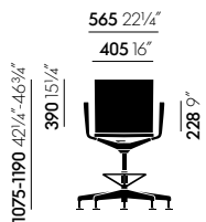
.04 Counter, Counterstuhl, mit Armlehnen
