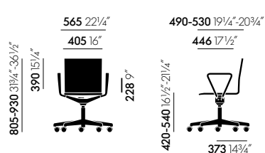
.04, Atelierstuhl, mit Armlehnen
