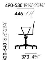
.04, Atelierstuhl, mit Armlehnen
